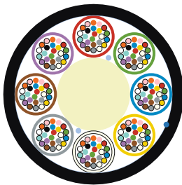
8x24-200µm
