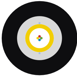
1x4 E9/125
