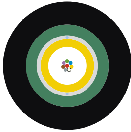
1x8 E9/125
